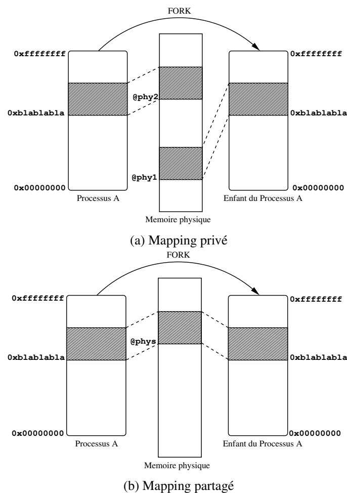
FIGURE 4.1 – Différence entre mapping privé et partagé après un fork
