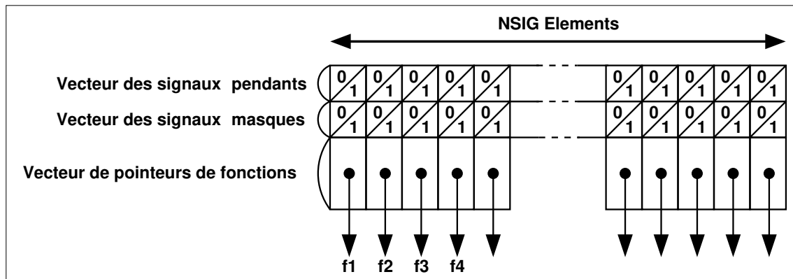
FIGURE 6.2 – Structures de données pour la gestion des signaux classiques.
