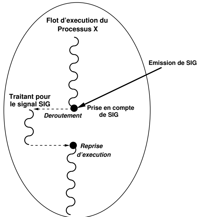
FIGURE 6.1 – Déroutement d'un processus vers un traitement de signal
